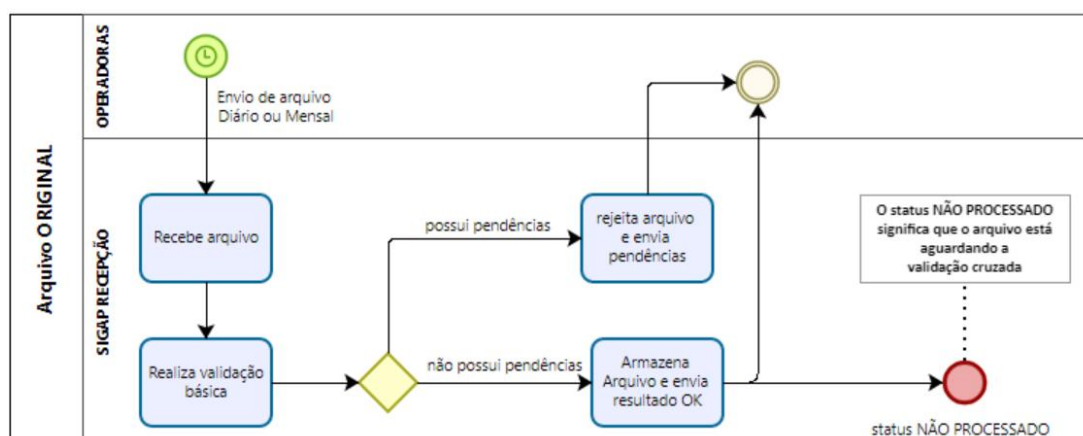
Figura 4 - Fluxo da validação básica - ARQUIVO ORIGINAL
