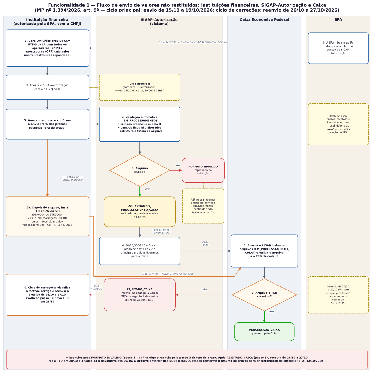
Figura 1 – Fluxo de upload do arquivo de valores não restituídos (IF / SIGAP-Autorização / Caixa / SPA e Banco Central)
